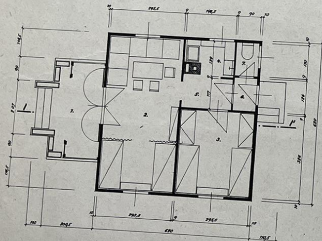
PŮDORYS
