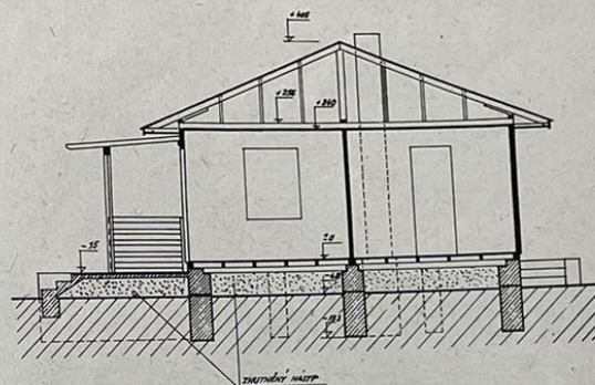
ŘEZ 1-1'
